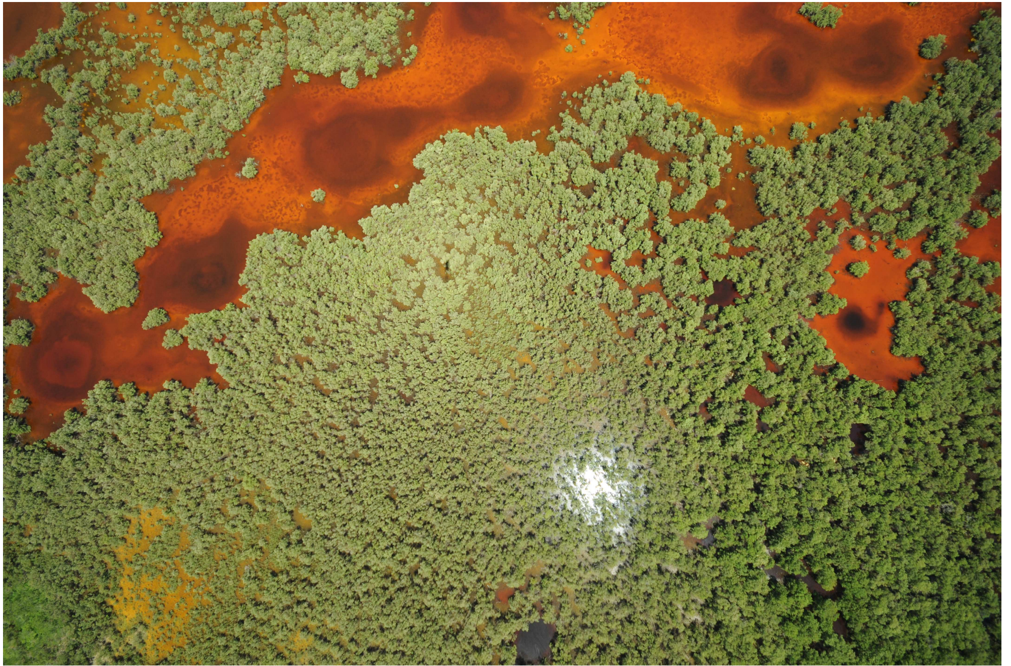
Fig. 4. Manglares de Peténes, Yucatán. CONABIO – SEMAR / J. Díaz (2008). Fotografía aérea vertical.
