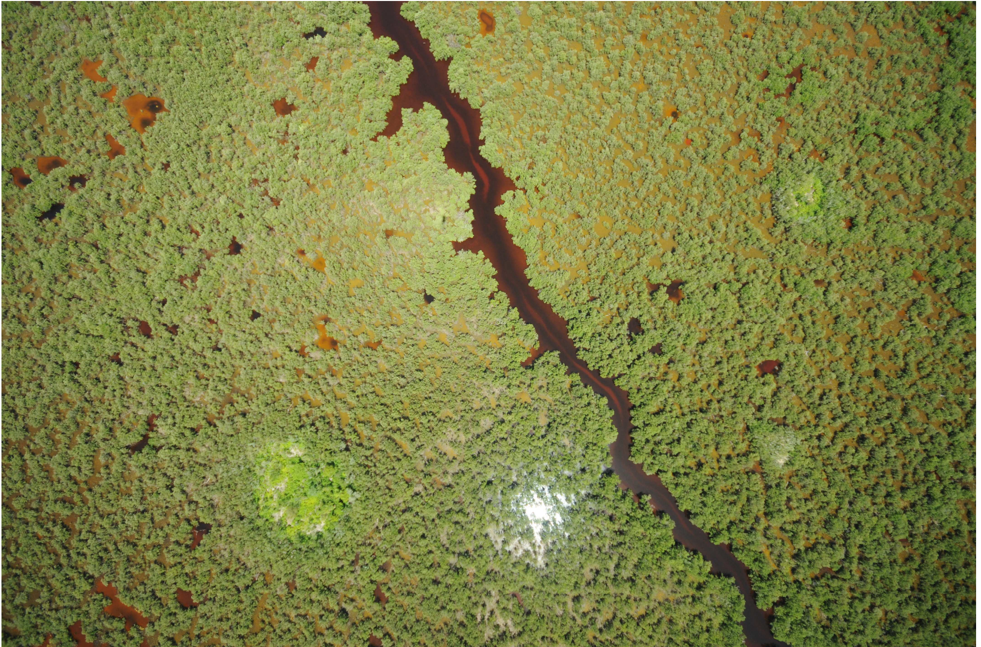
Fig. 1. Manglares de Peténes, Yucatán. CONABIO – SEMAR / J. Díaz (2008). Fotografía aérea vertical.
